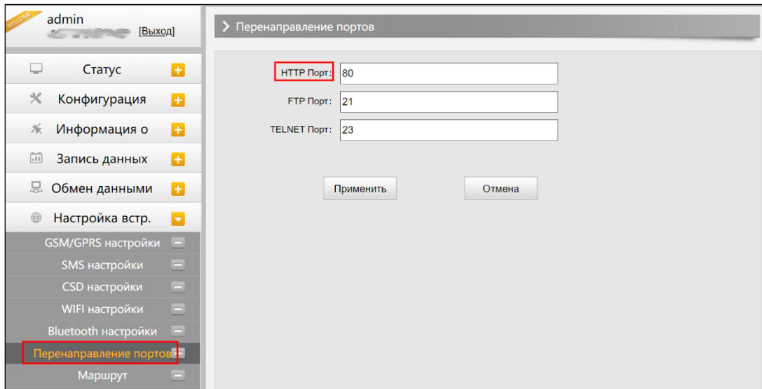
Веб-интерфейс, вкладка Настройки встр. GSM-Перенаправление портов
