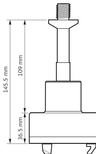
Адаптер GRT146 - установка на Штатив
